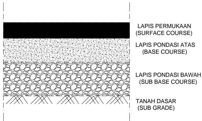
Gambar 2.13. Lapis Perkerasan Lentur
