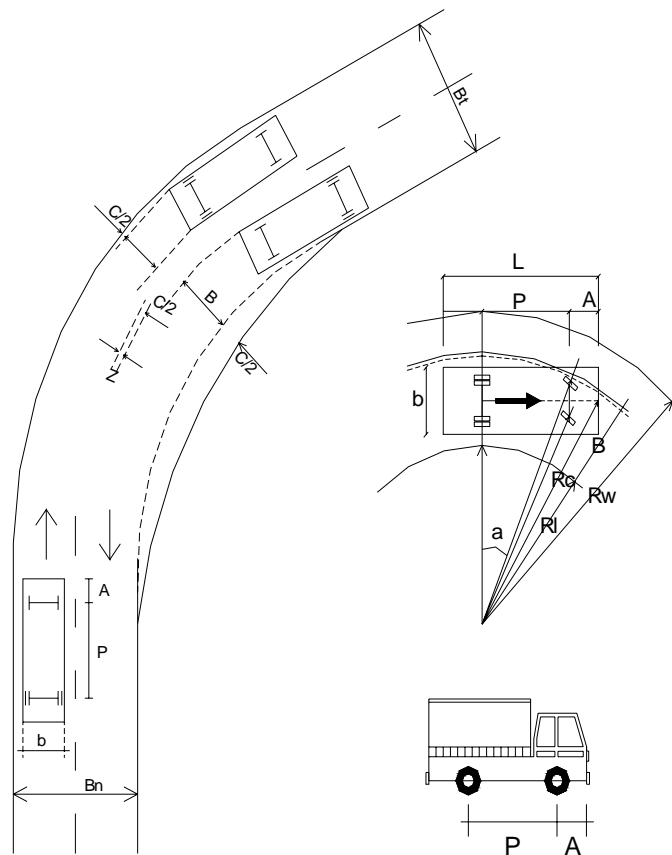
Gambar 2.4. Pelebaran Perkerasan Pada Tikungan
