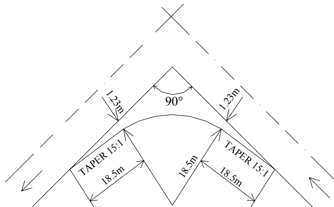
Gambar 2.10b. Rancangan Minimum Untuk Truk Unit Tunggal Dan Bis
