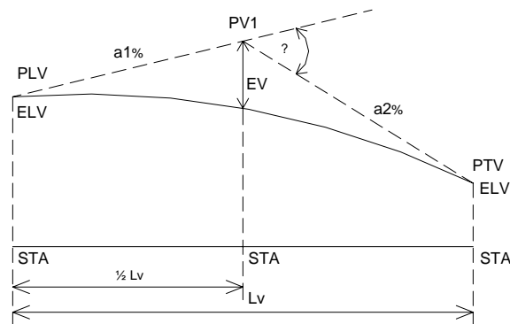
Gambar 2.11. Alinyemen Vertikal Cembung
