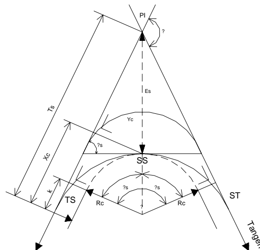
Gambar 2.3. Lengkung Spiral – Spiral
