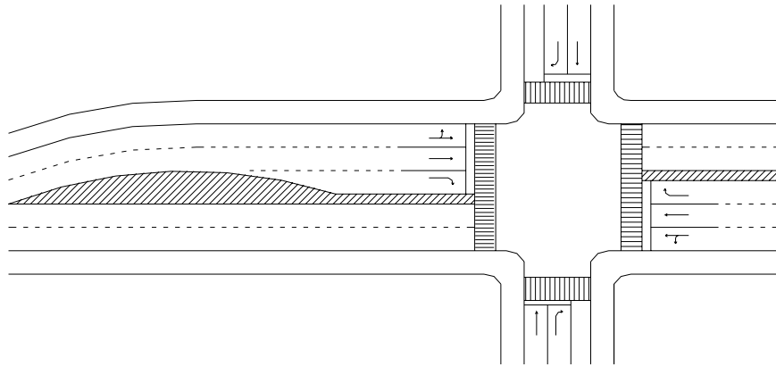
Gambar 2.7. Lajur Utama Digeser Untuk Lajur Belok-Kanan (Lajur Utama Dipersempit , Sedangkan Lebar Total Diperbesar)
