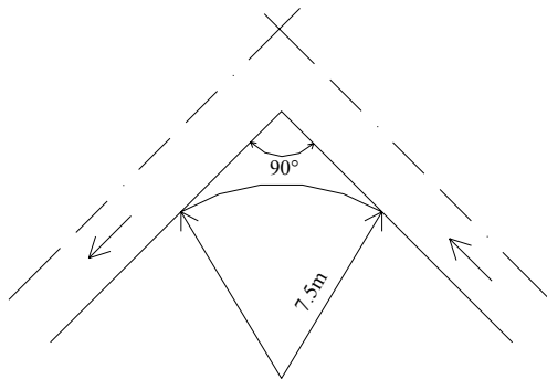
Gambar 2.10b. Rancangan Minimum Untuk Truk Unit Tunggal Dan Bis
