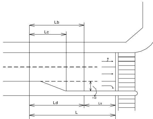
Gambar 2.6. Jalur Belok Kanan (Jalur Meian)
