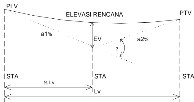
Gambar 2.12. Alinyemen Vertikal Cekung
