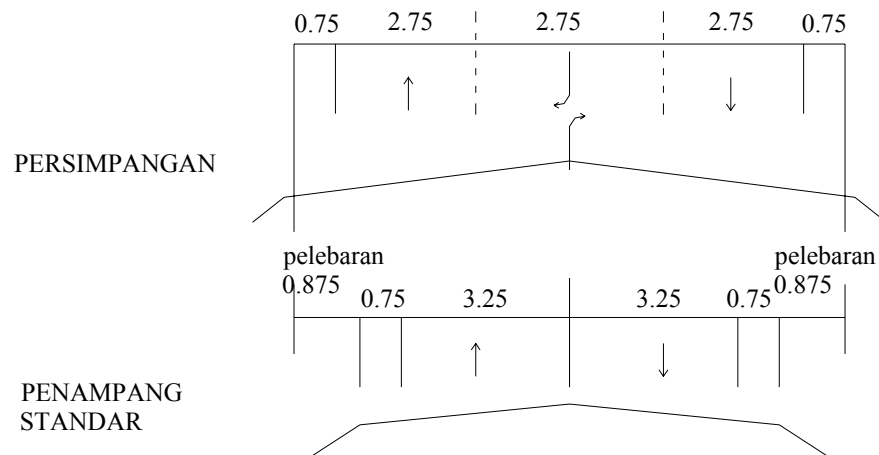
Gambar 2.9. Contoh Penyusunan Kembali Penampang Pada Persimpangan
