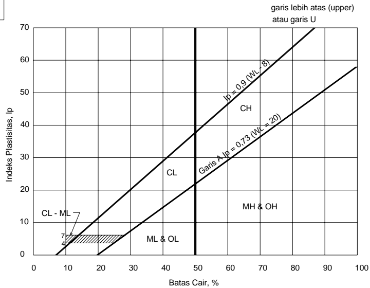
Grafik. 2.1. Bagan A (bagian plastisitas) dalam sistem USC
