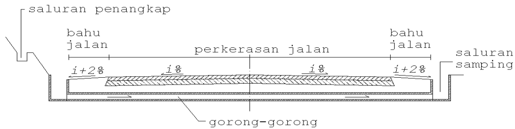
Gambar 2.14. Sistem Drainase Permukaan
