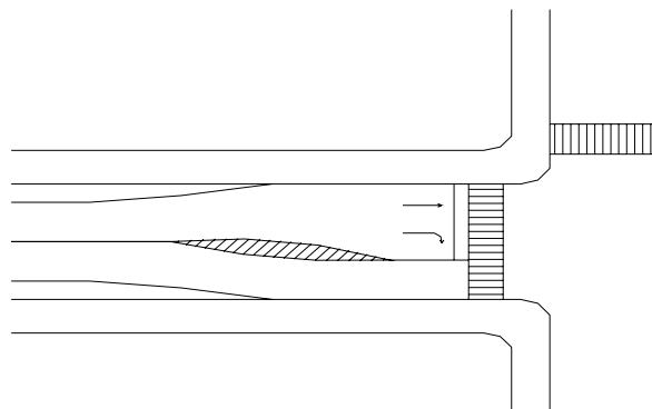
Gambar 2.8. Lajur Utama Digeser Yang Digeser Dan Diperlebar Untuk Ruang Belok-Kanan
