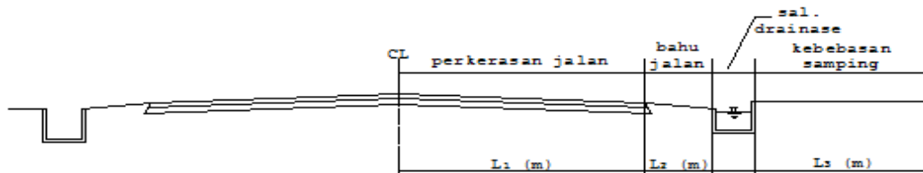
Gambar 2.15. Batas-Batas Daerah Pengaliran
