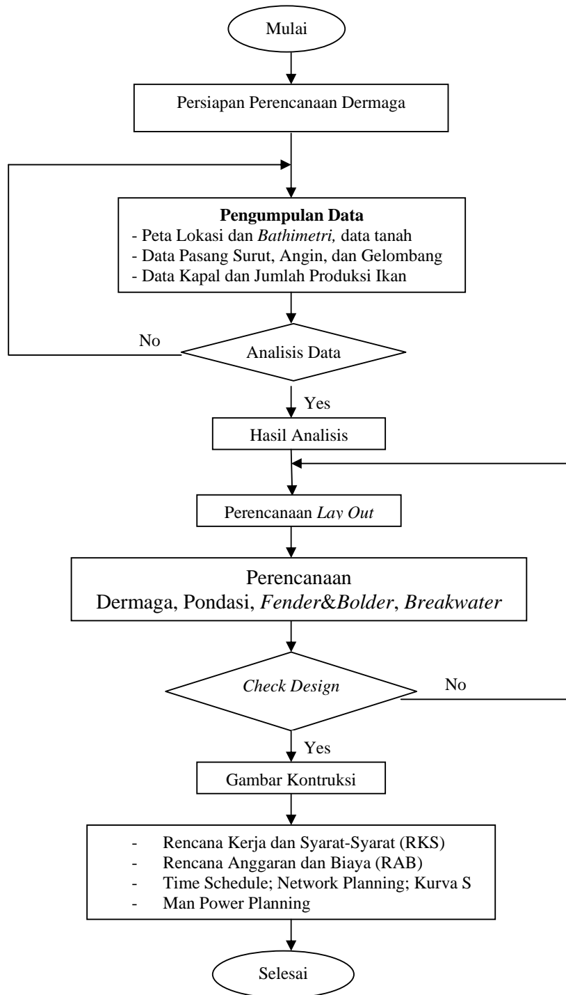
Gambar 4.1. Bagan Alir Perencanaan Dermaga
