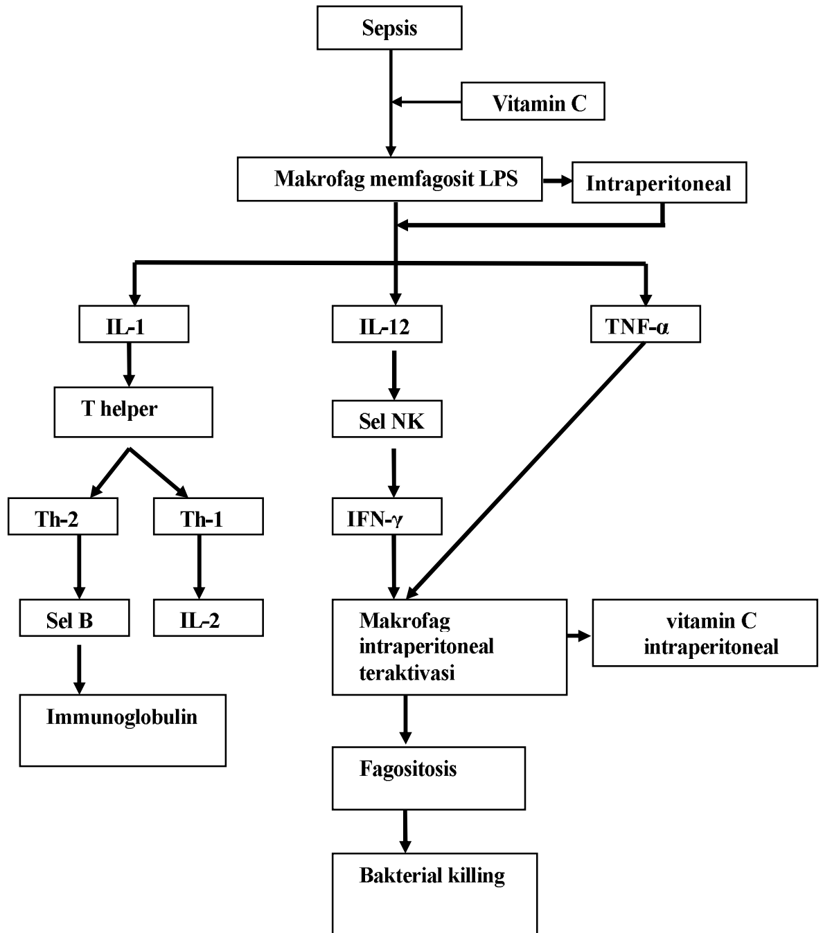
Gambar 5. Kerangka teori
