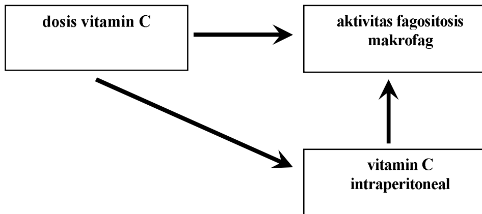
Gambar 6. Kerangka konsep
