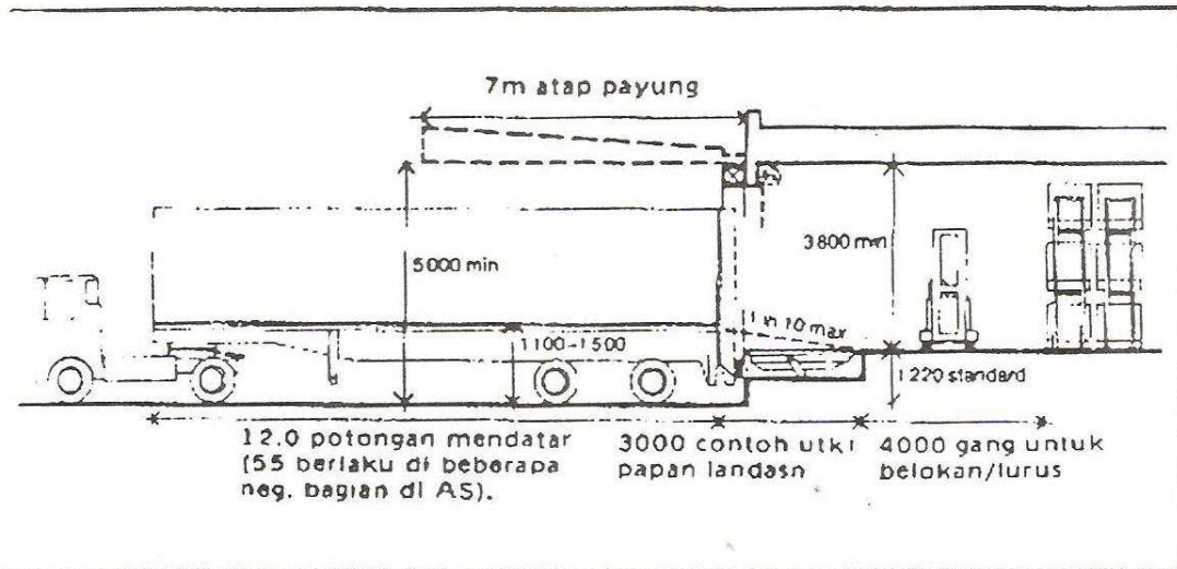
2. Gambar potongan panggung bongkar-muat yang diperlengkapi atap penangkap energi matahari: atap payung (titik-titik) hanya diperlukan bila tidak terdapat atap tambahan.
