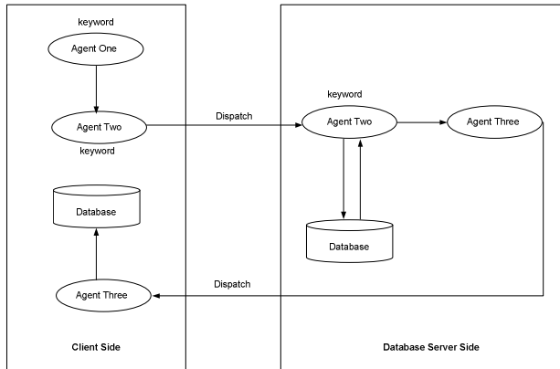
Gambar 4 Arsitektur sistem pencarian buku
