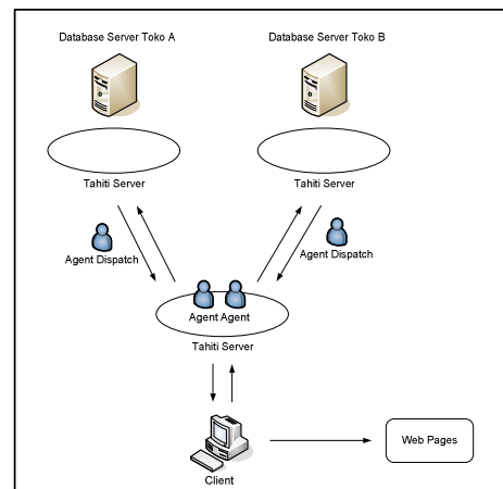
Gambar 3 Topologi sistem pencarian buku
