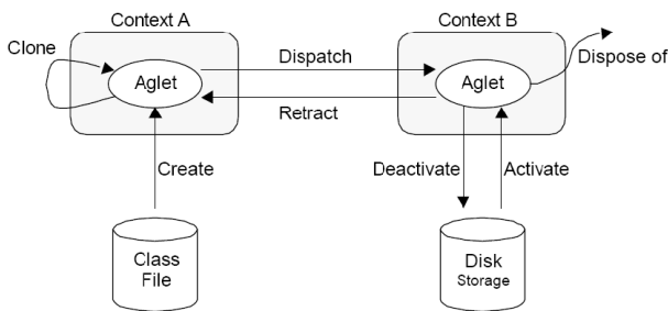
Gambar 2 Siklus hidup Aglet
