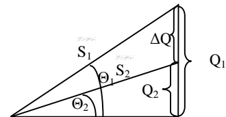
Gambar 4.1 Segitiga daya contoh perhitungan koreksi faktor daya
