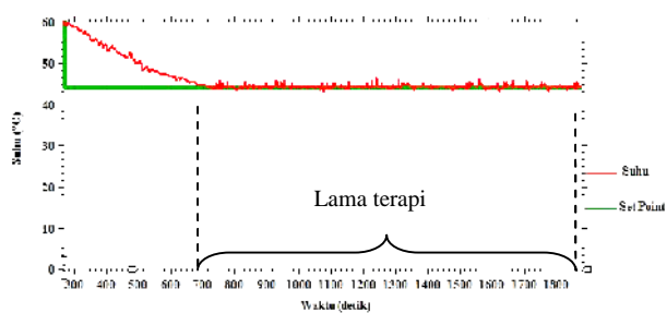
Gambar 4.18 Respon sistem kendali suhu dengan referensi 44 C dengan kondisi awal 65 C.
