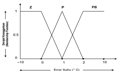
Gambar 8 Fungsi keanggotaan error level.
