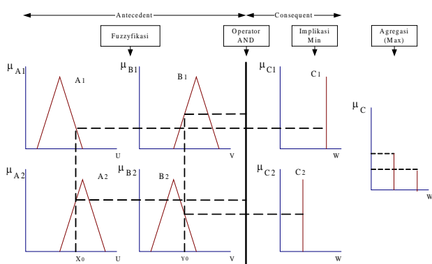
Gambar 4 Proses pengambilan keputusan metode Sugeno.
