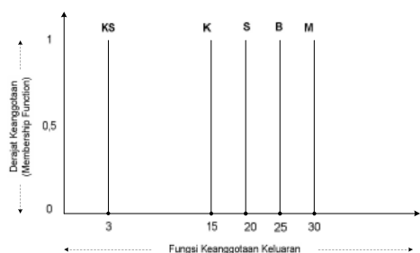
Gambar 10 Fungsi keanggotaan keluaran konstanta K_p .
