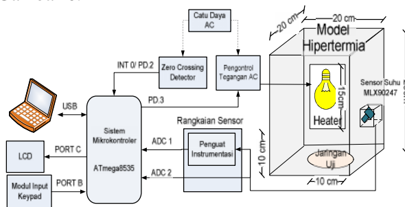
Gambar 6 Diagram blok perancangan perangkat keras.
