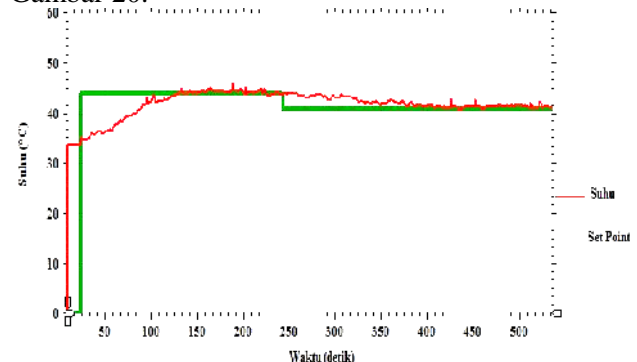
Gambar 20 Respon sistem pada referensi turun.
