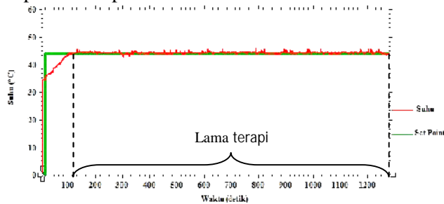
Gambar 4.17 Respon sistem kendali suhu dengan referensi 44 C dengan kondisi awal 34,5 C.
