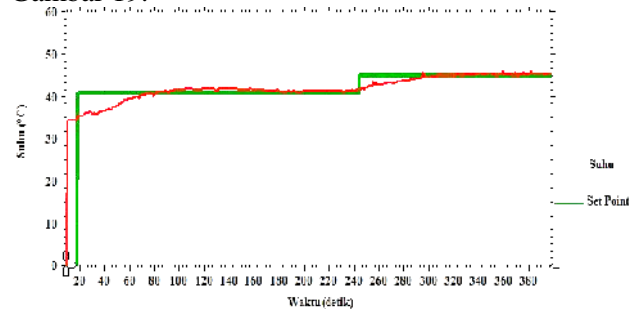
Gambar 19 Respon sistem pada referensi naik.
