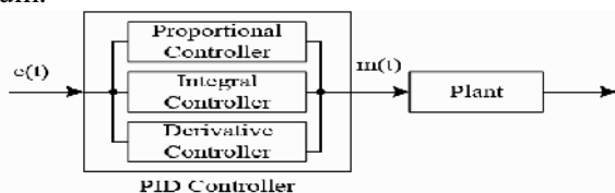
Gambar 1 Diagram blok pengendali PID secara umum.
