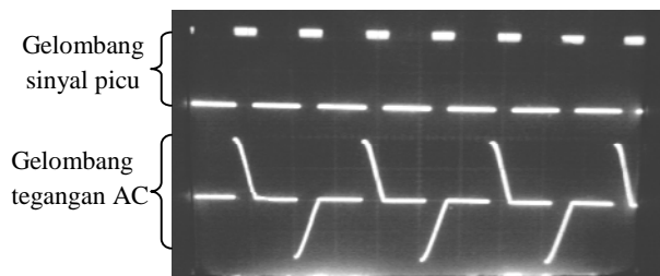
Gambar 13 Sinyal picu dan tegangan beban untuk C_o = 0\% .
