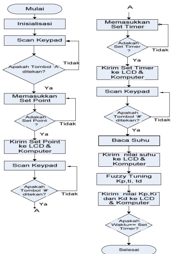
Gambar 7 Diagram alir sistem
