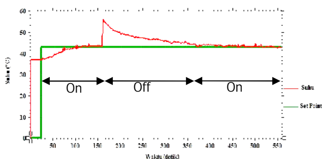
Gambar 21 Respon sistem terhadap gangguan.
