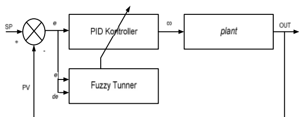
Gambar 5 Kontroler PID yang diadaptasi oleh Fuzzy sebagai tuning.
