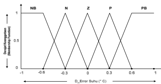
Gambar 9 Fungsi keanggotaan d_error level.
