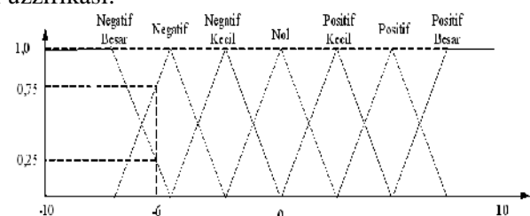
Gambar 3 Proses Fuzzifikasi.
