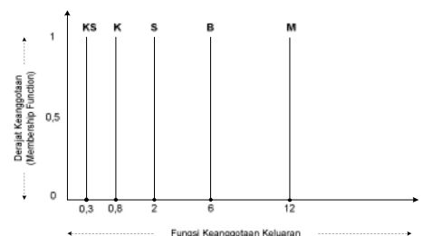
Gambar 12 Fungsi keanggotaan keluaran konstanta K_d .
