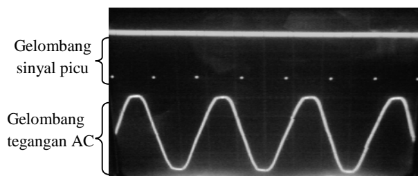
Gambar 15 Sinyal picu, tegangan beban untuk C_o = 100\% .
