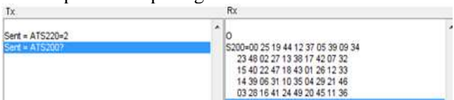
Gambar 17 Hopping table untuk register S220=2 (all band)
