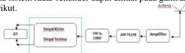
Gambar 3 Sistem Transmisi Data
