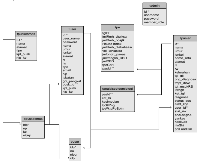
Gambar 6 Perancangan Basisdata
