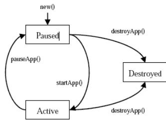
Gambar 3 Siklus MIDlet
