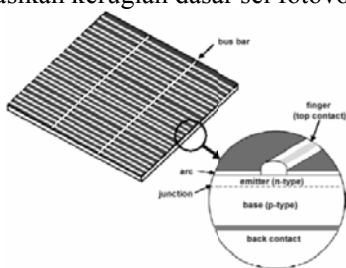
Gambar 1 Struktur sel fotovoltaik silicon crystalline [15]
