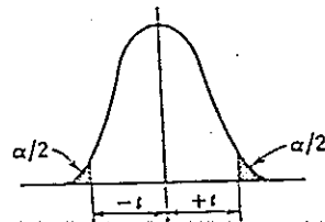
Sebaran t
