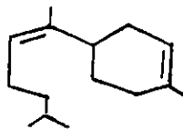
\delta -Kadinen
