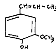
Isoeugenol
