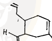
Akoron
