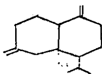
Kalamen
