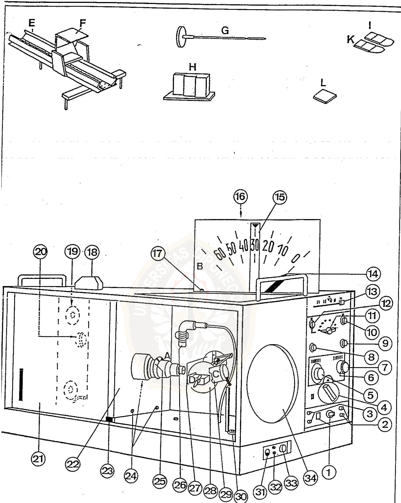
Fig. 2: Röntgen-Grundgerät, 42 kV (554 90). Lieferumfang und Beschreibung der Bedienelemente s. Seite 3ff.
