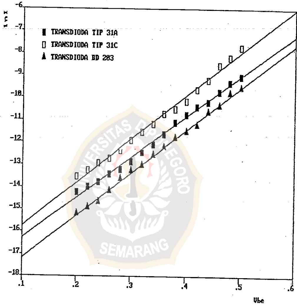
KARAKTERISTIK U/I PADA t = 50\text{ C}
