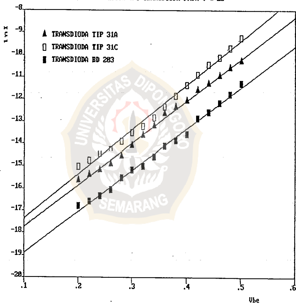
KARAKTERISTIK V/I TRANSDIODA PADA t = 25
