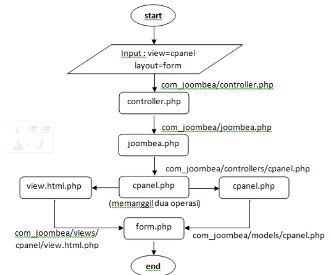
Gambar 15 Alur kerja pengujian white box
