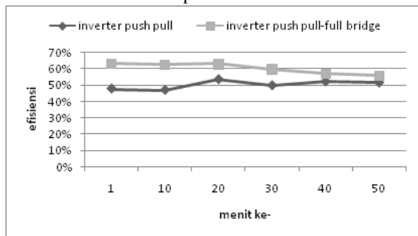
Gambar 30 Grafik perbandingan inverter push pull dan inverter push pull-full bridge pada beban motor pompa air
