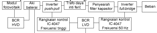
Gambar 8 Diagram blok perancangan
