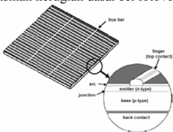
Gambar 1 Struktur sel fotovoltaik silicon crystalline [15]
