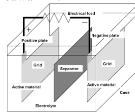
Gambar 4 Komposisi sel baterai [2]
