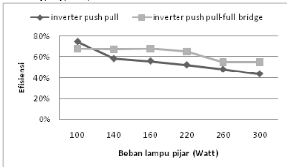
Gambar 29 Grafik perbandingan inverter push pull dan inverter push pull-full bridge pada beban lampu pijar
