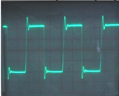
Gambar 19 Sinyal pemicuan trafo pulsa inti ferit 52.3 kHz (skala 1:1, V/div=5V, T/div=5us)
