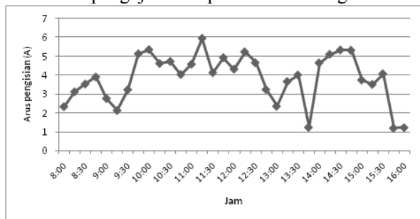
Gambar 26 Kurva hubungan tegangan dan arus pengisian dengan waktu pengisian hari Rabu
