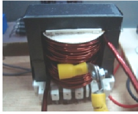
Gambar 13 Trafo daya inti ferit
