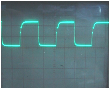
Gambar 18 Sinyal pemicuan IC 4047 52.3 kHz (skala 1:1, V/div=5V, T/div=5us)
