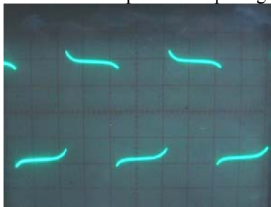
Gambar 21 Sinyal pemicuan trafo pulsa inti besi (skala 1:1, V/div=5V, T/div=5ms)
