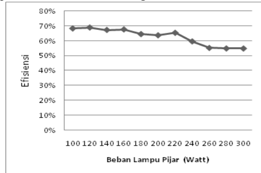
Gambar 27 Kurva hubungan pembebanan lampu pijar terhadap efisiensi
