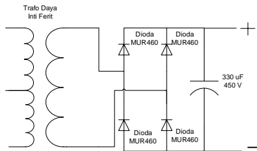
Gambar 14 Rangkaian penyearah gelombang penuh
