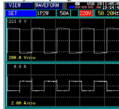
Gambar 24 Gelombang keluaran tegangan (atas) dan arus (bawah) beban lampu pijar
