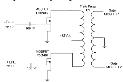
Gambar 12 Rangkaian driver dan trafo pulsa inti ferit
