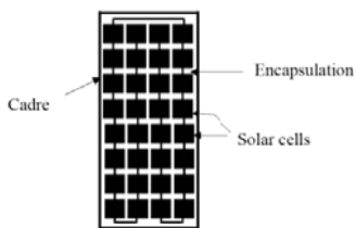
Gambar 2 Konstruksi modul fotovoltaik [15]
