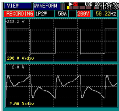
Gambar 25 Gelombang keluaran tegangan (atas) dan arus (bawah) beban pompa air
