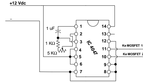
Gambar 16 Rangkaian Osilator frekuensi 50 Hz
