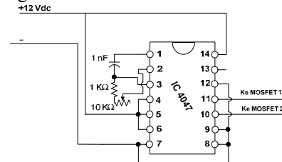
Gambar 11 Rangkaian osilator frekuensi tinggi
