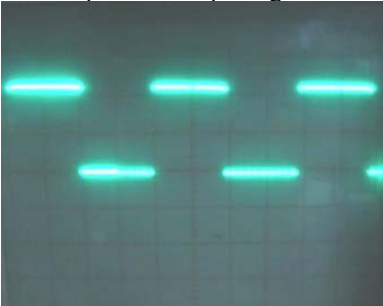
Gambar 20 Sinyal pemicuan IC 4047 frekuensi 50 Hz (skala 1:1, V/div=5V, T/div=5ms)
