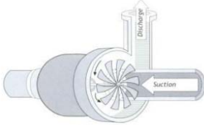
Gambar 7 Skema cara kerja motor pompa air [11]
