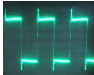
Gambar 22 Gelombang keluaran trafo daya inti ferit (skala 1:100, V/div=1V dan T/div=5us)
