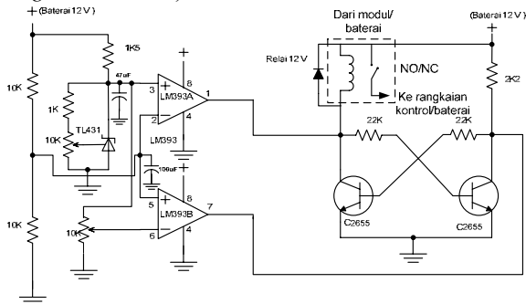
Gambar 9 Rangkaian HVD dan LVD
