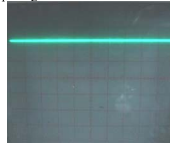
Gambar 23 Gelombang keluaran penyearah full bridge (skala 1:100, V/div=1V dan T/div=5ms)
