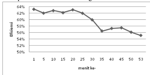
Gambar 28 Kurva hubungan pembebanan motor pompa air terhadap efisiensi hari Rabu
