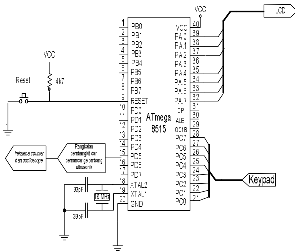
Gambar 4.3 Bentuk rangkaian pengujian mikrokontroler dengan menggunakan rangkaian pembangkit dan pemancar gelombang ultrasonik.
