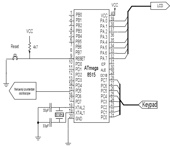
Gambar 4.1 Skema rangkaian pengujian sistem minimum mikrokontroler ATmega8515 dengan frekuensi counter dan oscilloscope .
