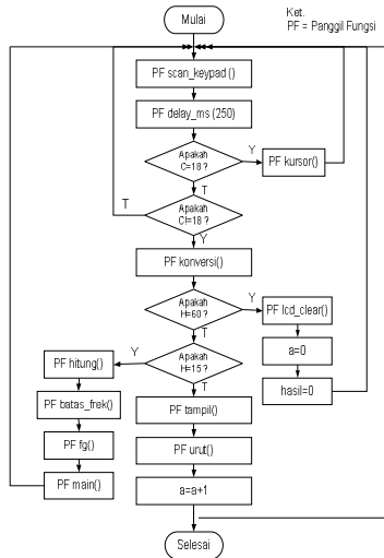
Gambar 3.6 Diagram alir program utama.
