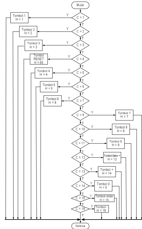
Gambar 3.8 Diagram alir fungsi konversi().
