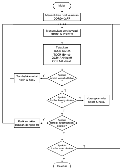
Gambar 3.7 Diagram alir fungsi generator().
