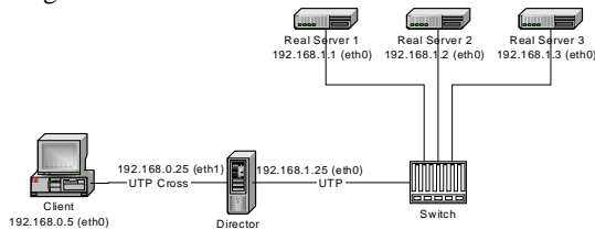
Gambar 3.2 Konfigurasi sistem komputer cluster
