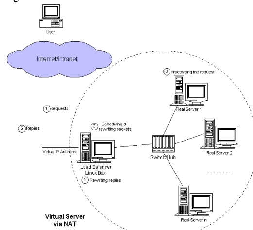
Gambar 2.9 Arsitektur virtual server via NAT
