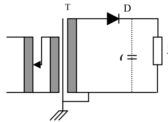
Gambar 2.1 Penyearah setengah gelombang
