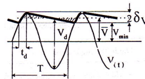
Gambar 2.3. Keluaran penyearah setengah gelombang dengan kondensator perata
