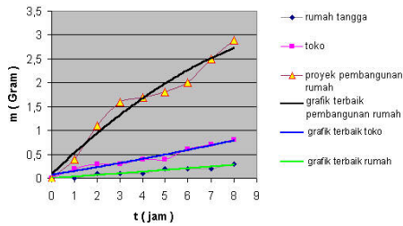
Gambar 4.3 Grafik hubungan massa debu dengan waktu sebelum menggunakan tegangan DC
