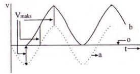
Gambar 2.5. Keluaran penyearah Villard
