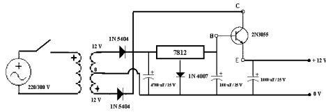
Gambar 3.4 Sumber tegangan 12 VDC
