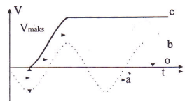
Gambar 2.7. Keluaran penyearah Greinacher
