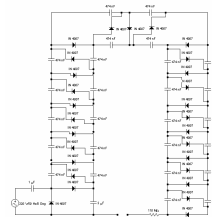
Gambar 3.2 Rangkaian pembangkit tegangan tinggi searah ( DC )
