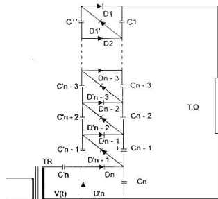
Gambar 2.8 Rangkaian Penyearah Kaskade
