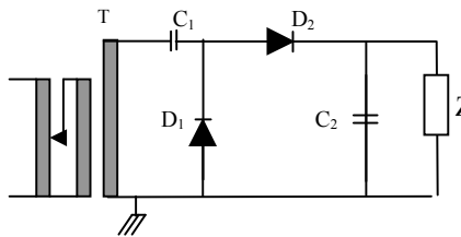
Gambar 2.6. Rangkaian penyearah Greinacher
