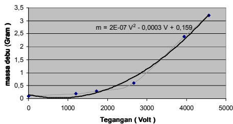
Gambar 4.1 Hubungan massa debu yang diendapkan dengan tegangan
