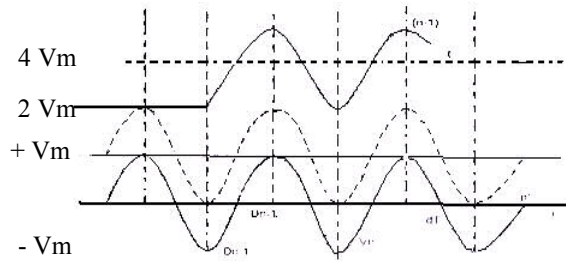
Gambar 2.9 Keluaran penyearah Kaskade
