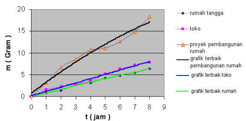
Gambar 4.4 Grafik hubungan massa debu dengan waktu setelah menggunakan tegangan tinggi DC
