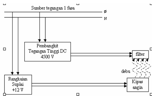
Gambar 3.1 Blok diagram alat
