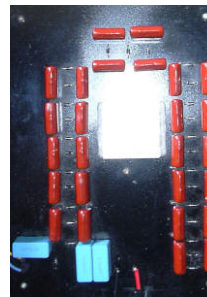
Gambar 3.3 Blok pembangkit tegangan DC yang telah dibuat
