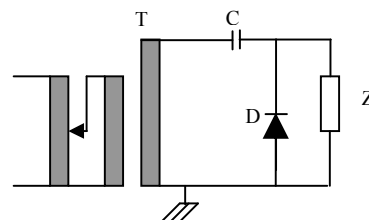
Gambar 2.4. Rangkaian penyearah Villard
