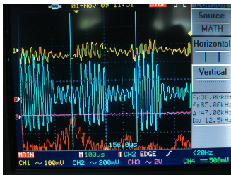
Gambar 4.9 Keluaran sinyal HPF 31 KHz.
