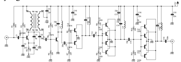
Gambar 3.7 Pemancar FM.
