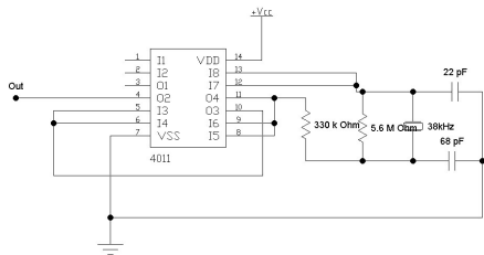
Gambar 3.3 Rangkaian osilator Kristal.
