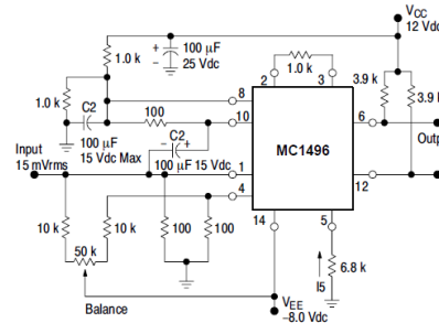
Gambar 3.13 Rangkaian pengali dua frekuensi.
