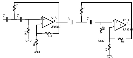
Gambar 3.14 Tapis pelolos tinggi 38 KHz.
