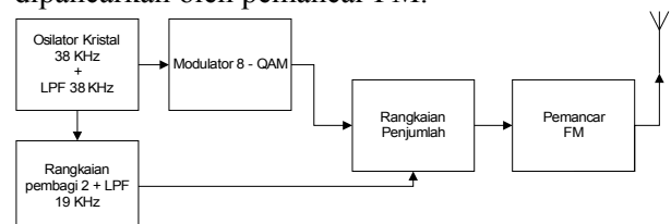
Gambar 3.2 Diagram blok sistem pada sisi pemancar.
