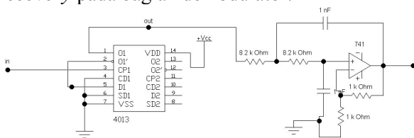
Gambar 3.5 Pembagi dua dan LPF 19 KHz.
