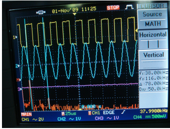
Gambar 4.2 Keluaran sinyal LPF 38 KHz.
