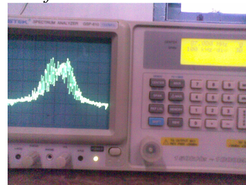
Gambar 4.6 Pengujian Daya yang dikeluarkan rangkaian FM.
