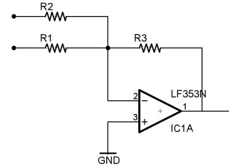
Gambar 3.6 Penjumlah sinyal.
