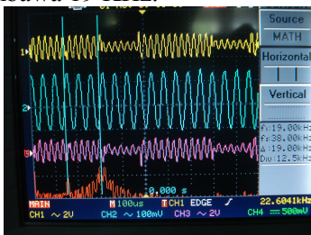
Gambar 4.5 Keluaran penjumlah.
