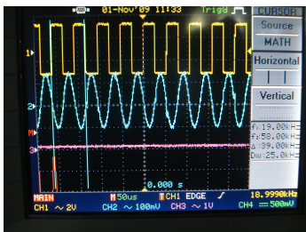
Gambar 4.4 Sinyal keluaran LPF 19 KHz.
