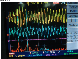
Gambar 4.11 sinyal keluaran pengganda frekuensi
