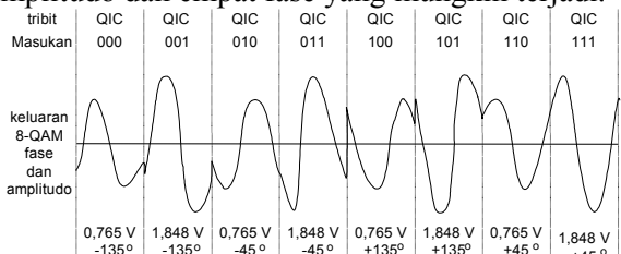
Gambar 2.2 Keluaran amplitudo dan fase terhadap waktu.
