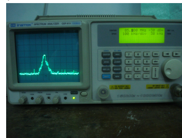
Gambar 4.7 Spektrum dalam ruangan dengan jarak 3 meter.
