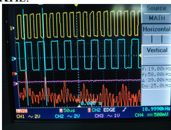
Gambar 4.3 Keluaran sinyal pembagi dua.
