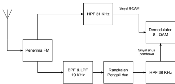
Gambar 3.9 Diagram blok sistem pada sisi penerima.
