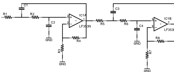
Gambar 3.12 Tapis pelolos rendah 19 KHz.
