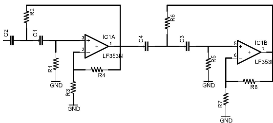
Gambar 3.10 Tapis pelolos tinggi 31 KHz.
