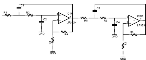
Gambar 3.4 Tapis pelolos bawah.
