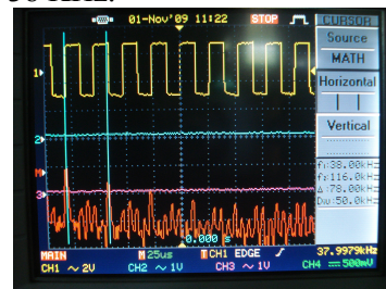
Gambar 4.1 Keluaran osilator kristal 38 KHz.
