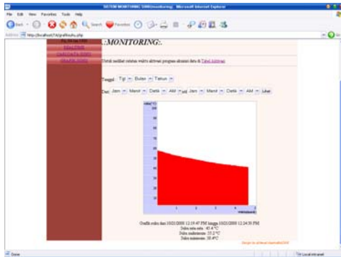
Gambar 4.7 halaman grafiksuhu.php .
