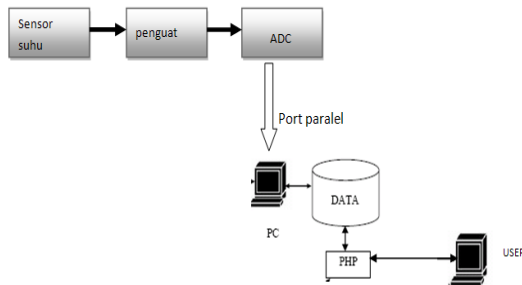
Gambar 3.1 Diagram blok sistem.
