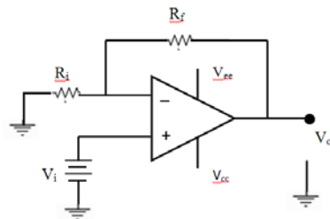
Gambar 2.1 Penguat tak membalik.
