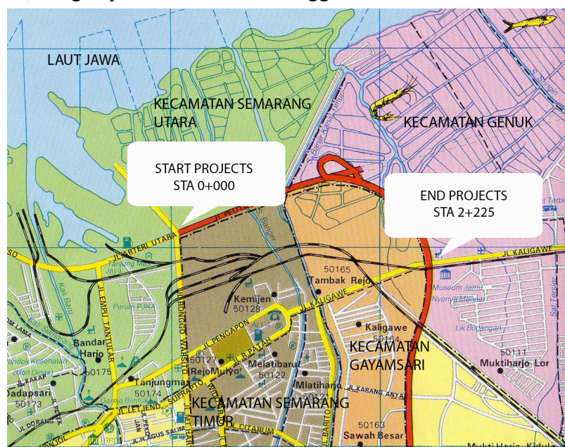
Gambar 1.1 Layout Jalur Arteri Utara Semarang
