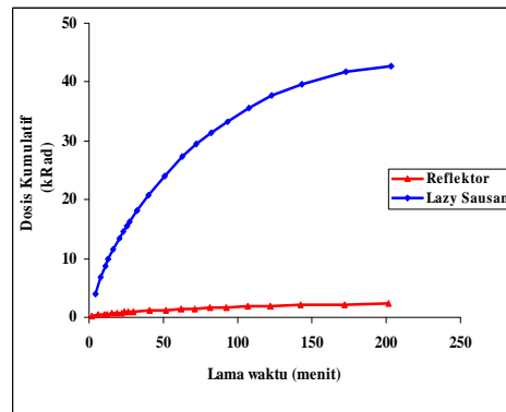
Gambar 5 Grafik dosis kumulatif pada dinding luar reflektor Reaktor Kartini
