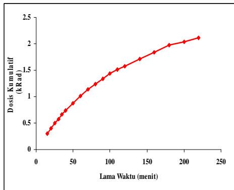
Gambar 4. Grafik dosis kumulatif pada dinding luar reflektor Reaktor Kartini
