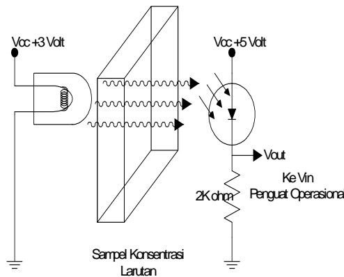
Gambar 2. Rangkaian Sensor
