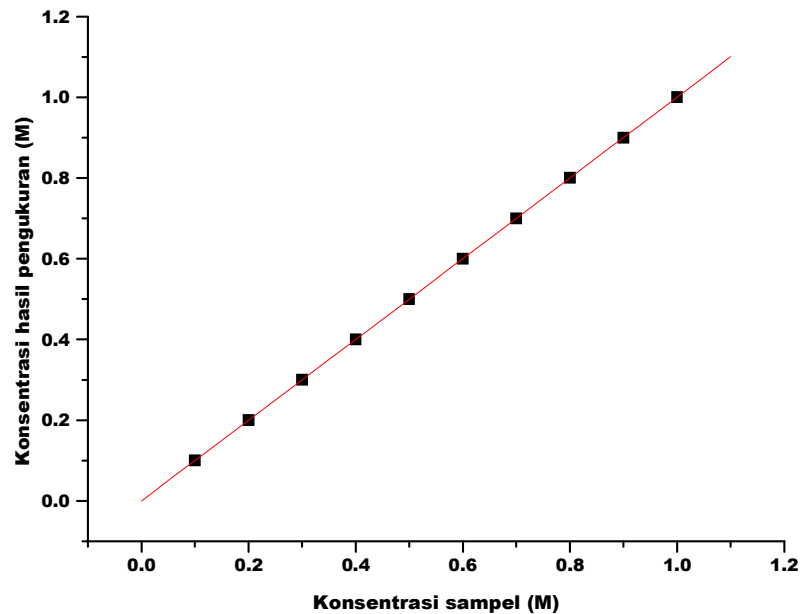
Gambar 8 Grafik hasil pengukuran sample
