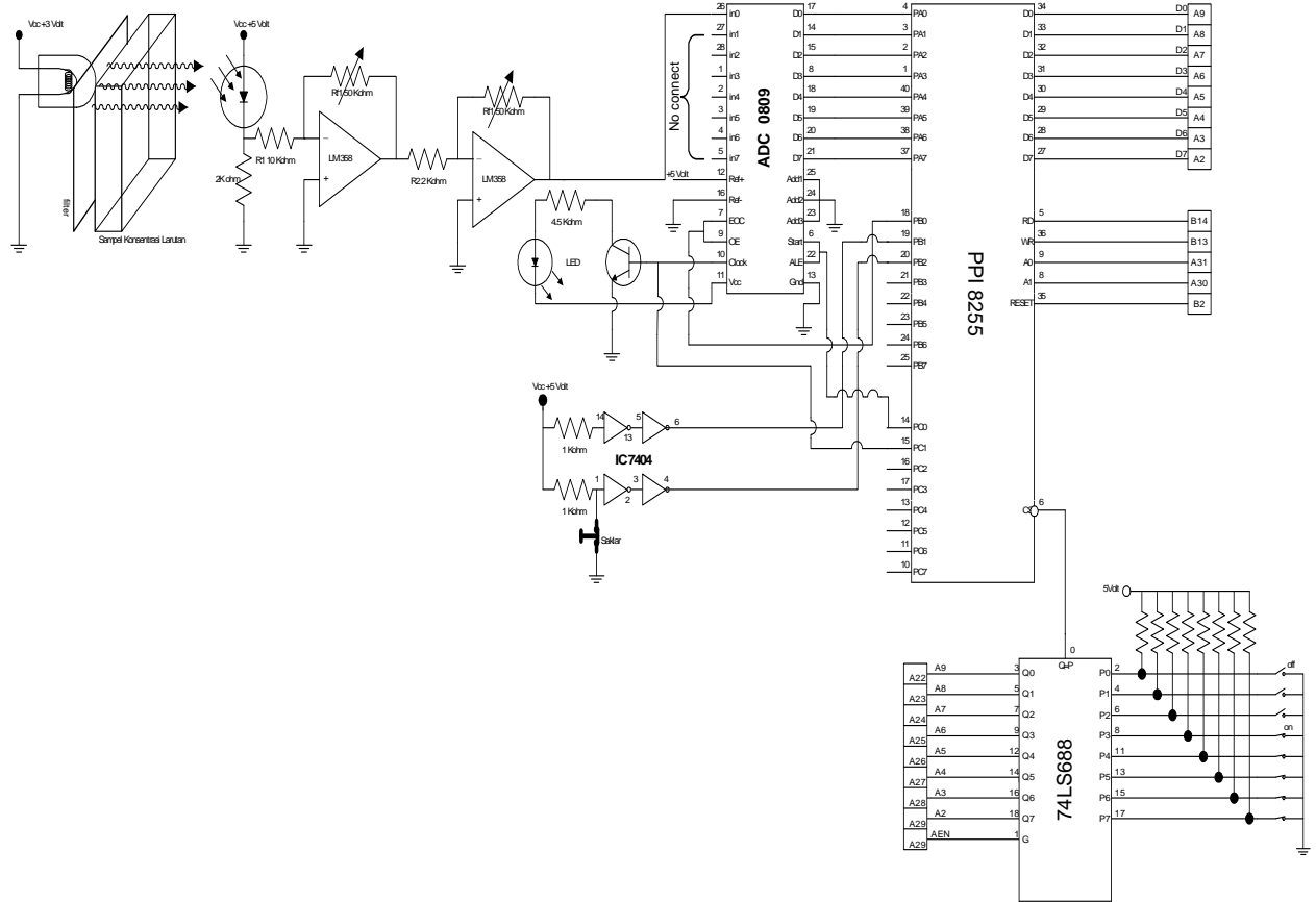
Gambar 5. Realisasi rangkaian sistem pengukur
