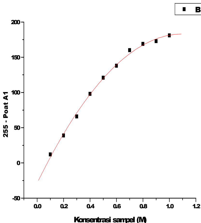
Gambar 6. Grafik hasil pengujian sistem
