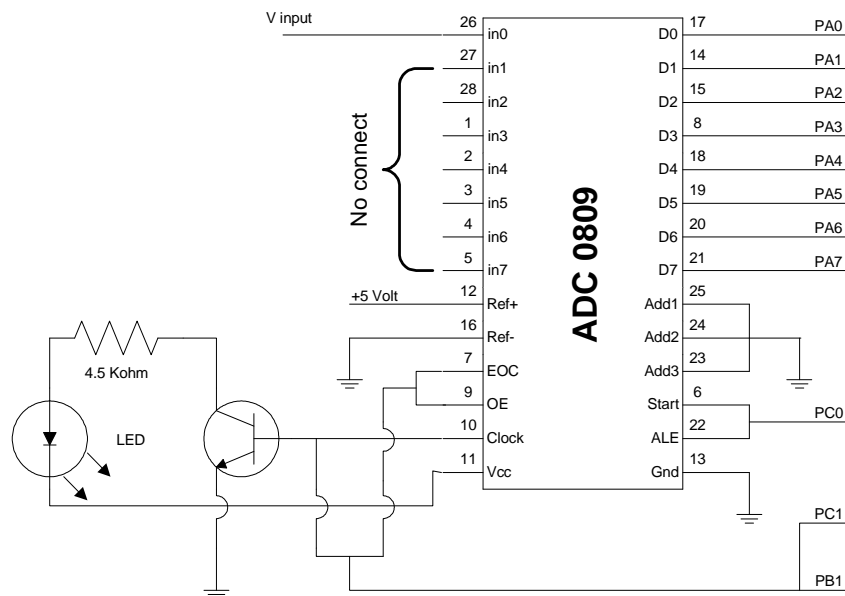
Gambar 3. Rangkaian pengubah sinyal analog ke digital
