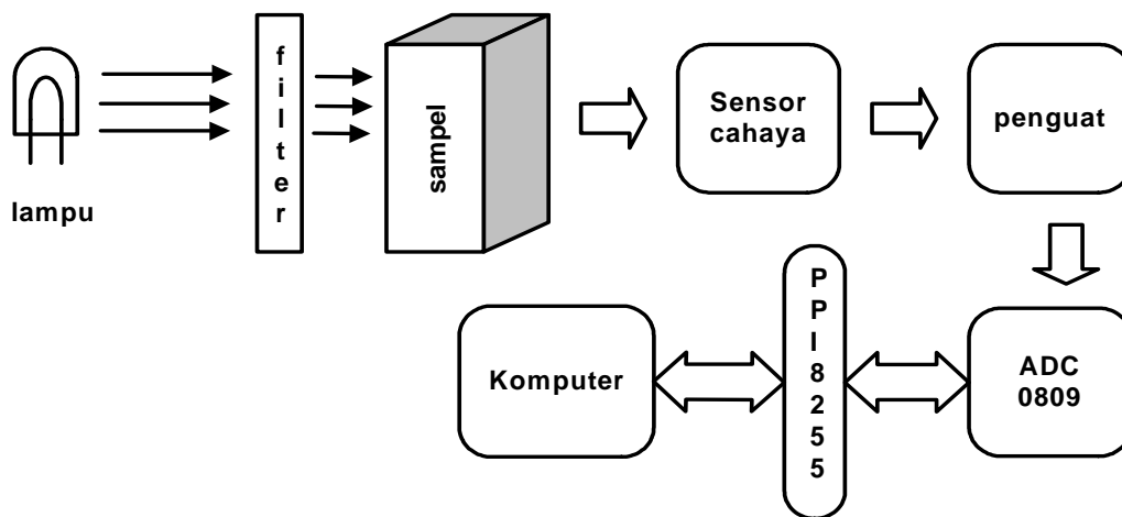
Gambar 1. Diagram Blok sistem
