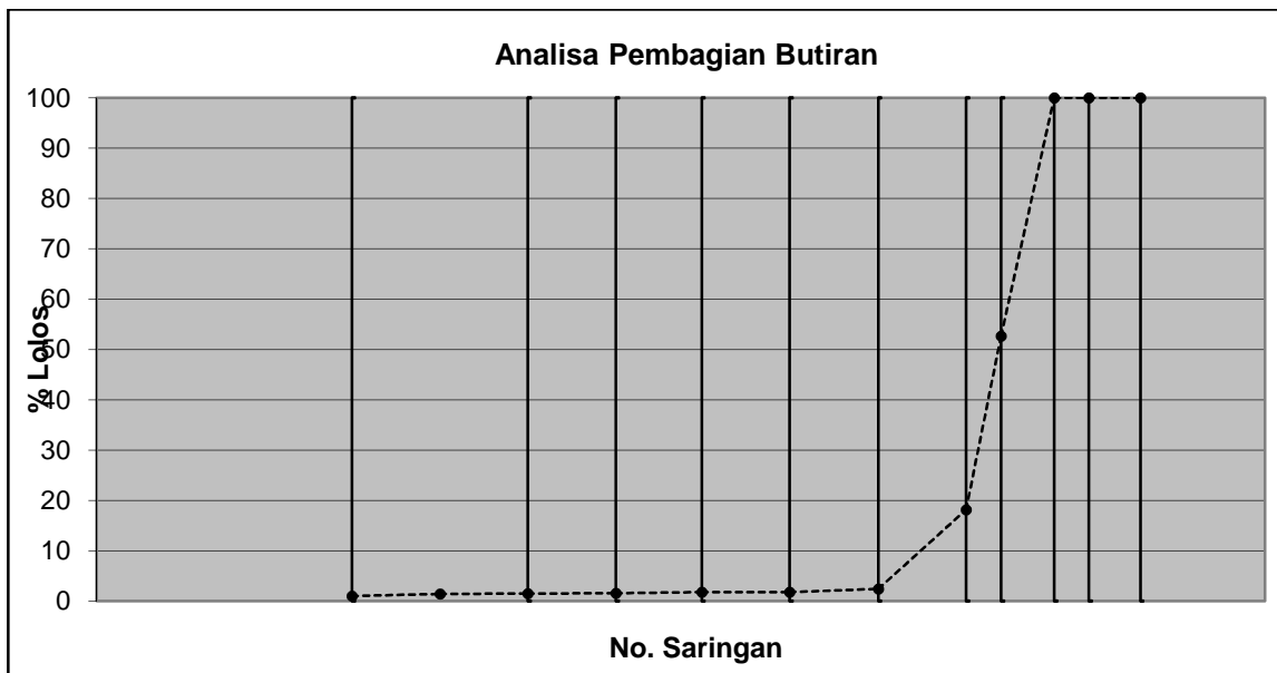
Gambar 1 Grafik Analisa Pembagian Butiran Batu Pecah ¾"
