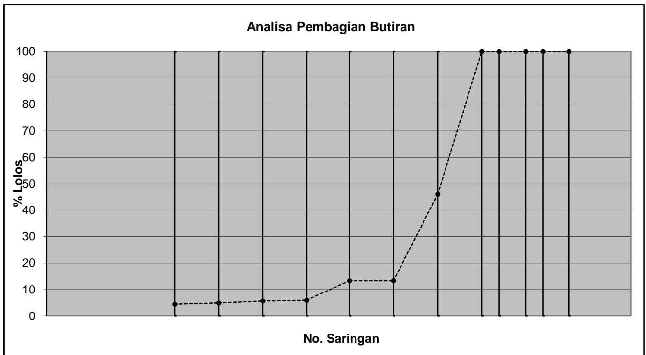
Gambar 2 Grafik Analisa Pembagian Butiran Batu Pecah 3/8''
