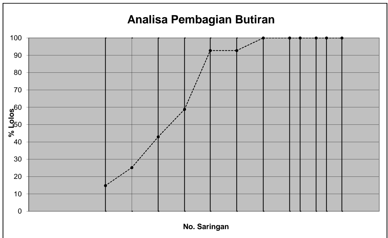
Gambar 4 Grafik Analisa Pembagian Butiran Pasir
