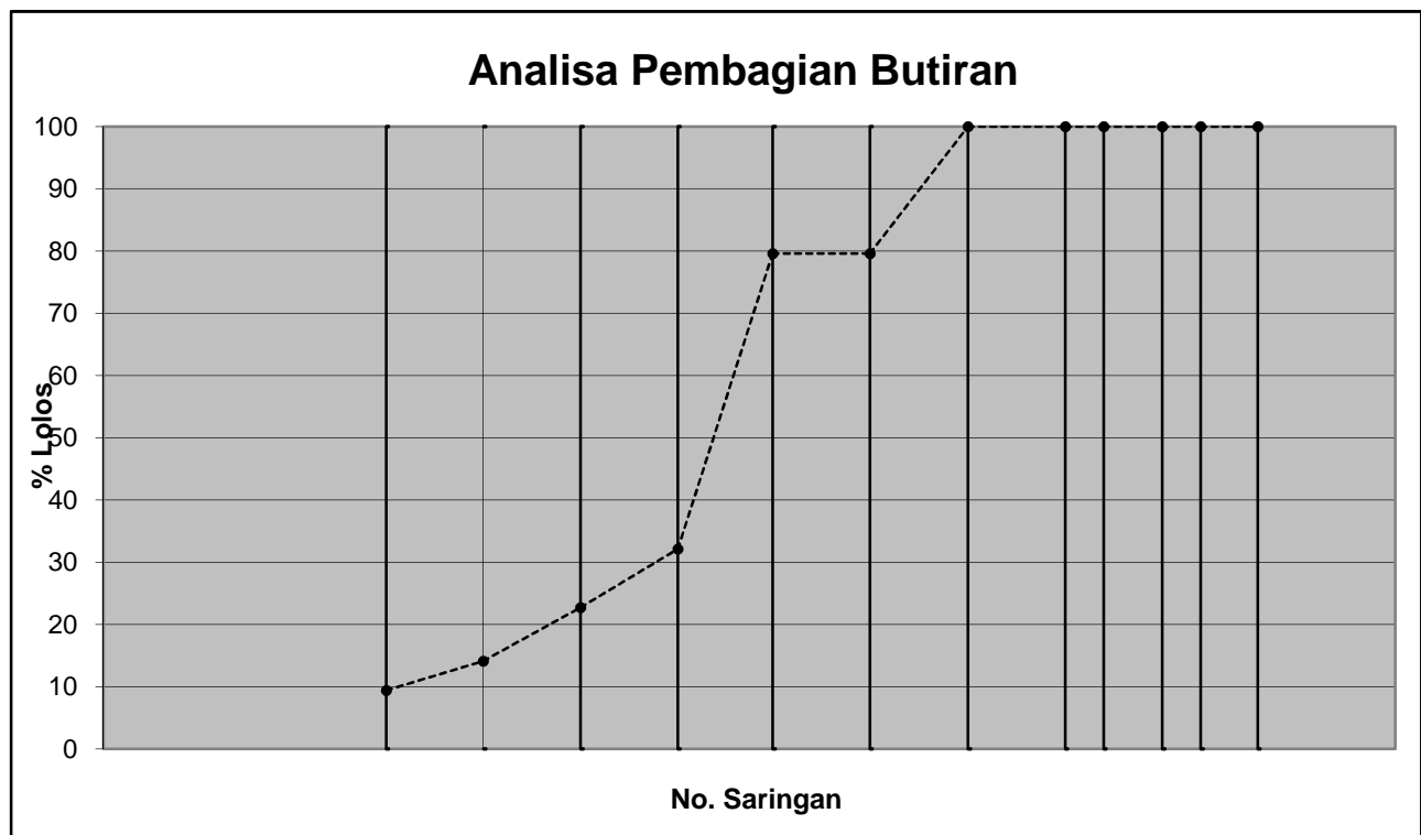
Gambar 3 Grafik Analisa Pembagian Butiran Abu Batu
