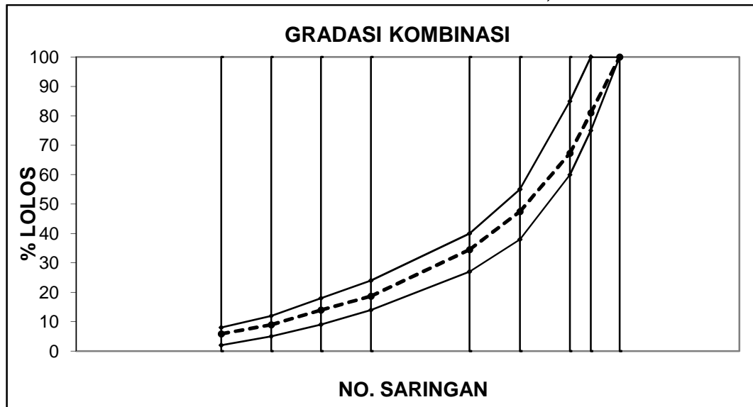
Gambar 5 Grafik Gradasi Kombinasi
