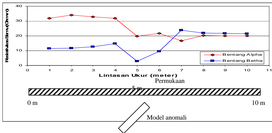
Gambar 2. Grafik respon anomali model konfigurasi persegi mapping dengan jarak elektroda ( a ) 1 m pada lintasan N 50 W
