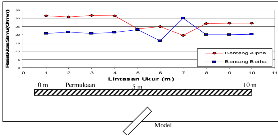
Gambar 1. Grafik respon anomali model konfigurasi persegi mapping dengan jarak elektroda ( a ) 1 meter pada lintasan N 40 W
