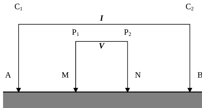
Gambar 2. Konfigurasi Schlumberger, MN adalah elektroda potensial, AB adalah elektroda arus, C 1 C 2 adalah arus yang terukur pada elektroda arus AB, P 1 P 2 adalah potesial yang terukur pada elektroda potensial MN [4]
