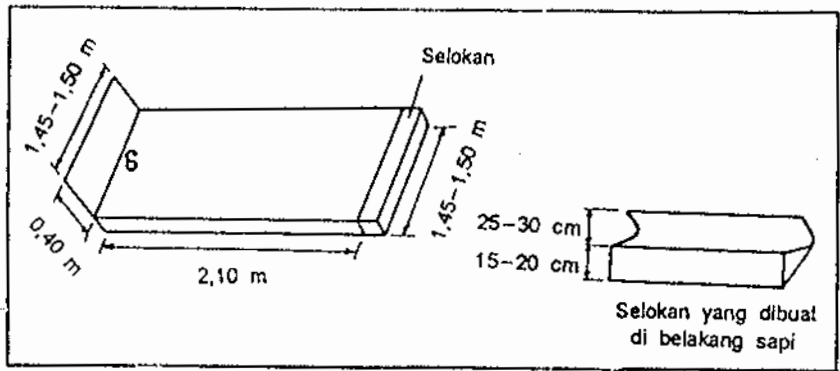
Gambar 15 : Ukuran kandang sapi
