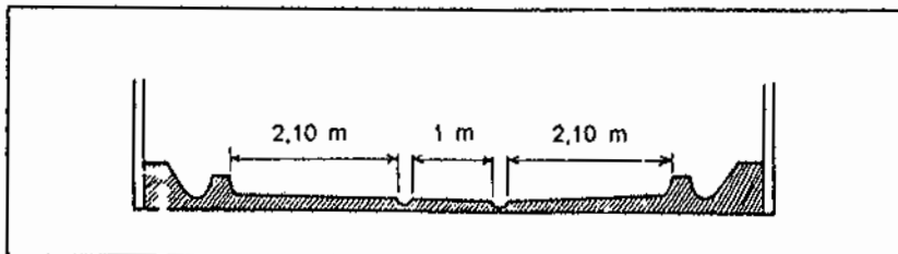
Gambar 14 : Penampang dasar kandang tipe ganda
