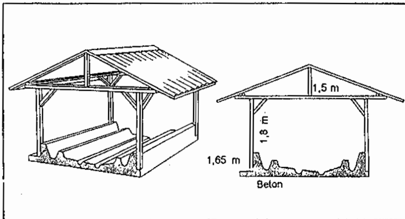
Gambar 13 : Kandang sapi tipe ganda
