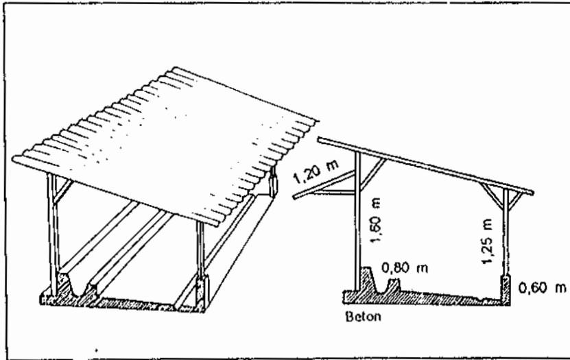
Gambar 12 : Kandang sapi tipe tunggal
