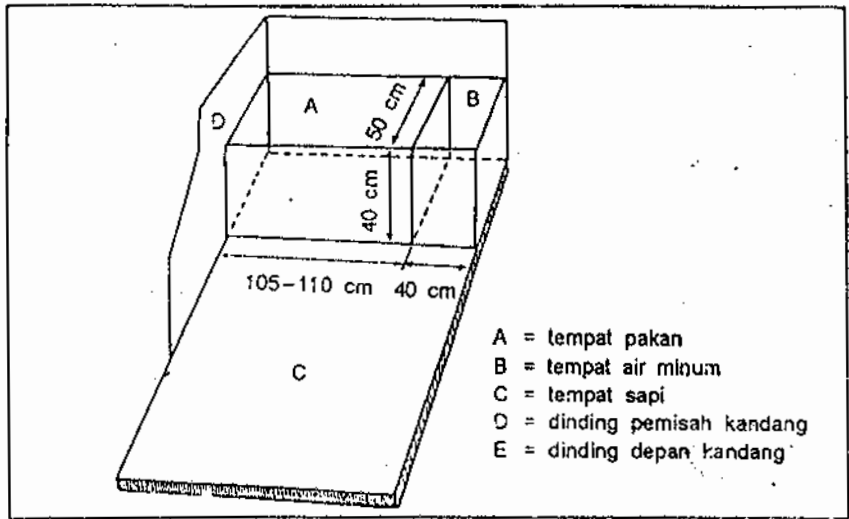
Gambar 16 : Tempat pakan dan minum
