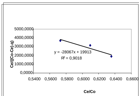
Gambar 10 Grafik Untuk Menentukan Isoterm BET (Karbon Aktif dari Plastik Ukuran 30-60 mesh)
