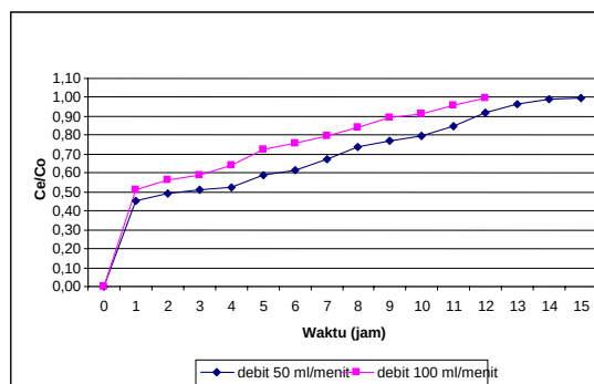
Gambar 11 Grafik Terobosan pada Kolom Kontinyu
