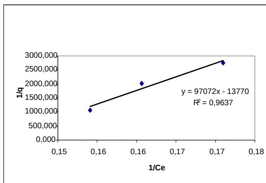
Gambar 8 Grafik Untuk Menentukan Isoterm Langmuir (Karbon Aktif dari Plastik Ukuran 30-60 mesh)
