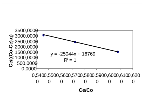
Gambar 9 Grafik Untuk Menentukan Isoterm BET (Karbon Aktif dari Plastik Ukuran 100-200 mesh)
