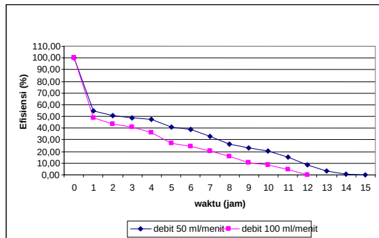
Gambar 12 Grafik Efisiensi pada Kolom Kontinyu
