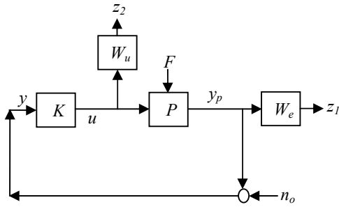
Gambar 4.2. Diagram blok dari Plant beserta bobot kontrol, bobot kinerja dan pengontrol
