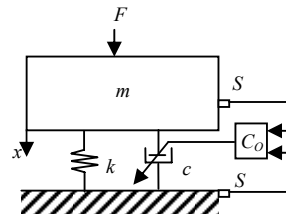
Gambar 4.1. Desain kontrol vibrasi semi aktif reaksi fixed point
