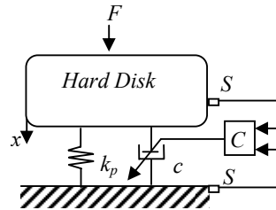
Gambar 4.3 Skema sistem proteksi Hard Disk dan pengontrolnya
