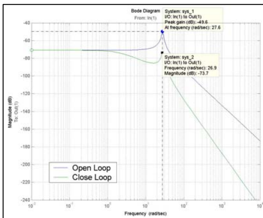
Gambar 4.4 Grafik Respon Frekuensi
