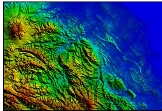
Gambar 7. DSM dari SRTM 30
