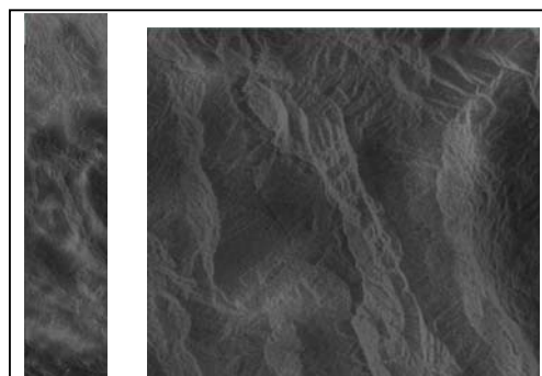
Gambar 4. Model Stereo Palsar (Pankromatik)
