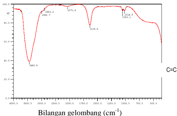
Bilangan gelombang ( \text{cm}^{-1} ) Gambar 5. Spektrum inframerah spiritus
