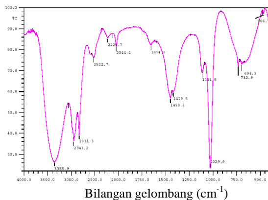
Gambar 7. Spektrum inframerah katalis
