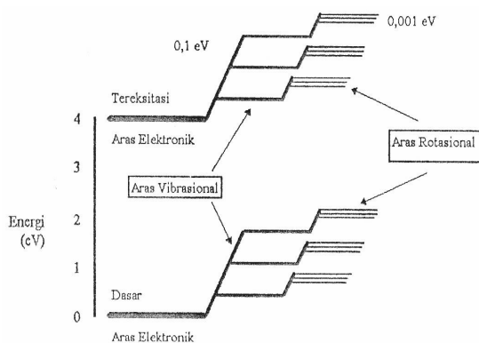
Gambar 1. Skema diagram tingkat energi molekul diatomik.
