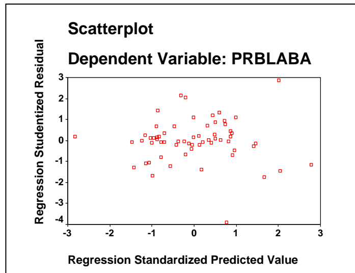
Gambar 4.5 Grafik Scatterplot Bank Non Devisa
