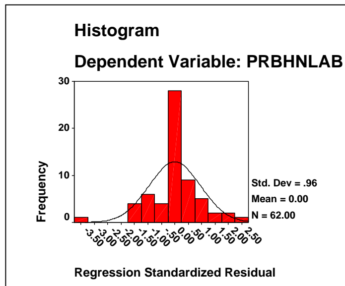
Grafik Histogram pada Bank Non Devisa (Data Ln)
