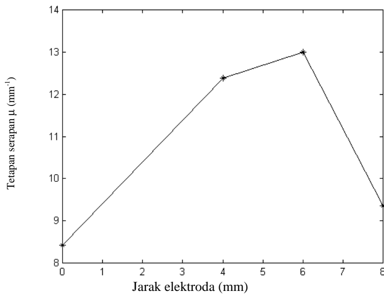
Gambar 4. Tetapan serapan ( \mu ) yang diperoleh pada beberapa nilai jarak elektroda. Waktu deposisi 30 menit, dengan tegangan elektroda sebesar 5 kV.
