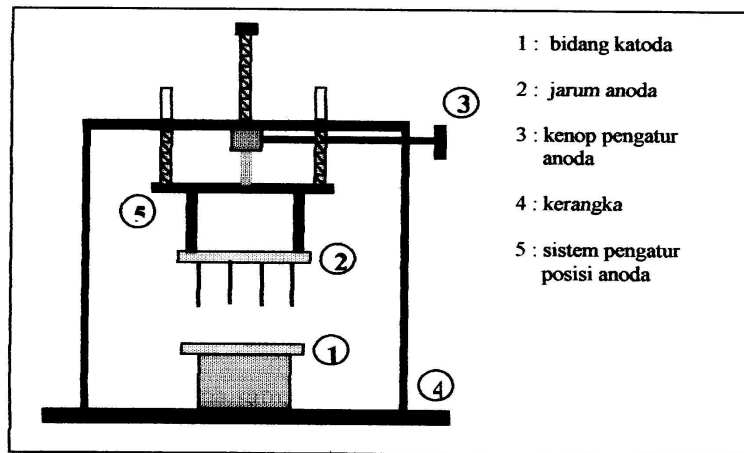
Gambar 1. Piranti pendeposisi metode lucutan korona
