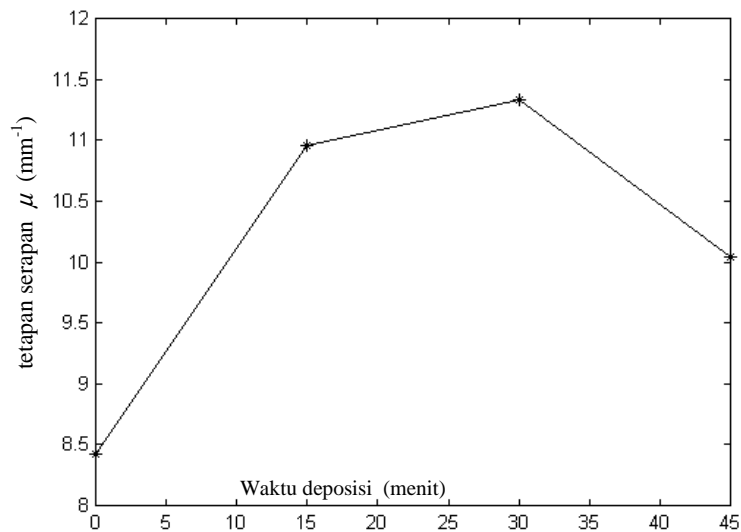
Gambar 2. Tetapan serapan ( \mu ) yang diperoleh pada beberapa nilai waktu deposisi. Tegangan elektroda yang digunakan 4,5 kV, dengan jarak elektroda sebesar 6 mm.
