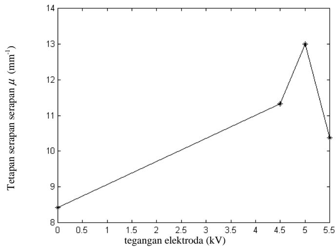
Gambar 3. Tetapan serapan ( \mu ) yang diperoleh pada beberapa nilai tegangan elektroda. Waktu deposisi 30 menit, dengan jarak elektroda sebesar 6 mm.
