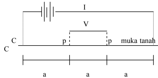
Gambar : pengaturan jarak elektroda pada metoda Wenner
