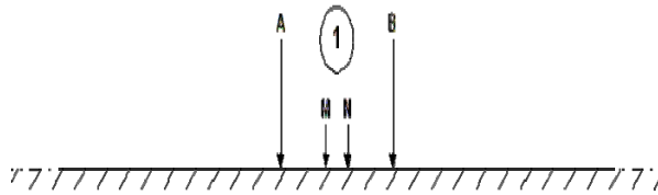
Gambar 5. Konfigurasi Metode Schlumberger (Anonim, 2007a).
