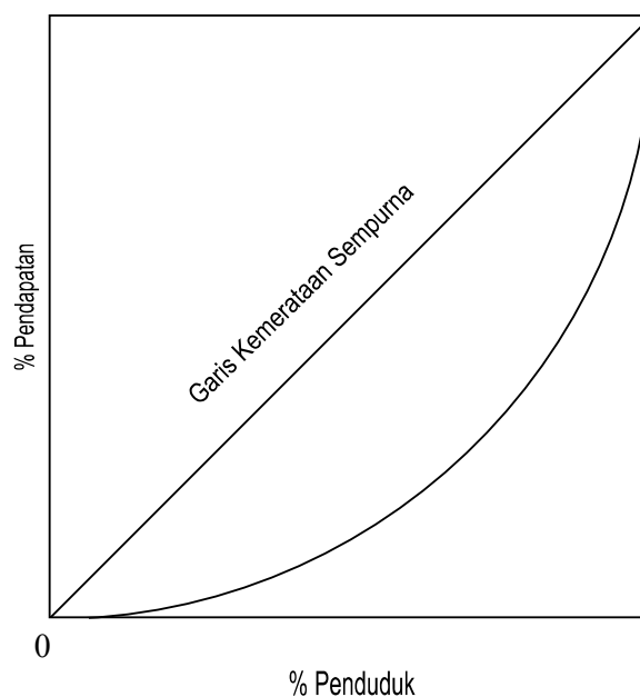
Gambar 2.3 Kurva Lorenz
