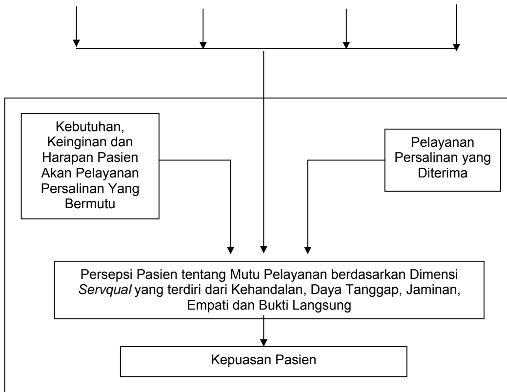
Gambar 2.1. Kerangka Teori
