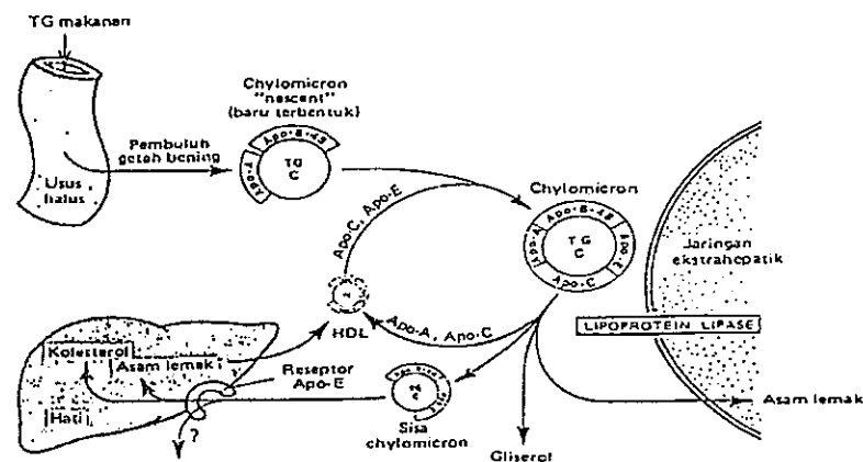
Gambar 1. Sistem eksogen sintesis lemak (Djokomoeljanto) 2
