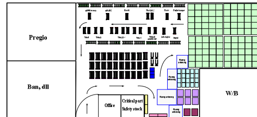
Gambar 4. Alternatif Layout II
