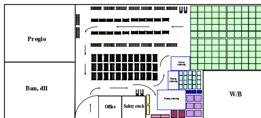
Gambar 3. Alternatif Layout I
